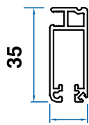
Profilo portarete
