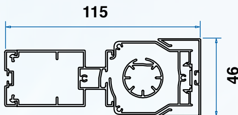
Profilo di copertura portamagnete Barramaniglia Cassonetto "U" di riscontro
